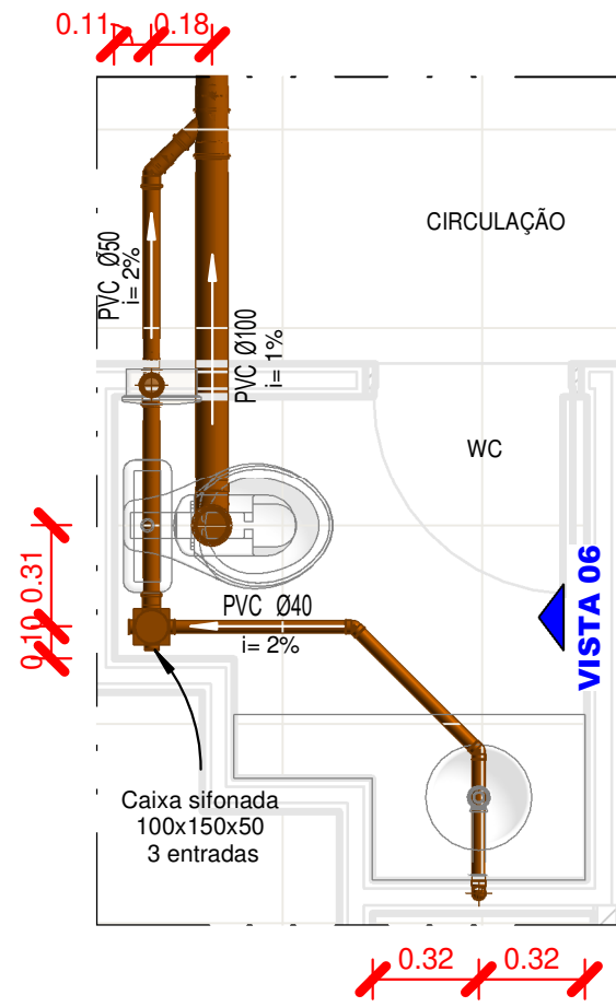
DETALHE 06 - ESGOTO 1 : 25
