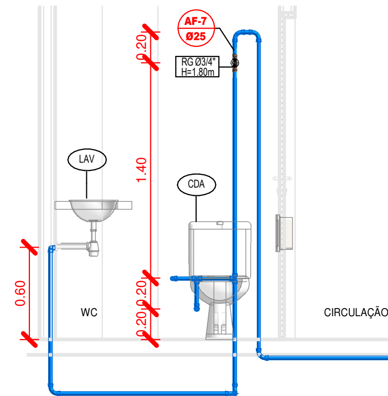
VISTA 06 - ÁGUA FRIA 1 : 25
