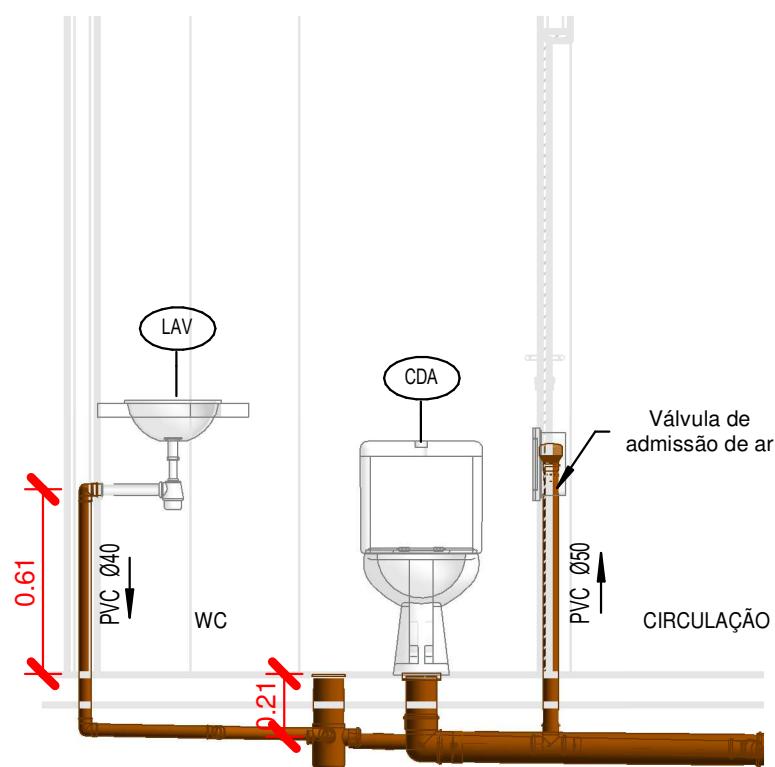
VISTA 06 - ESGOTO 1 : 25
