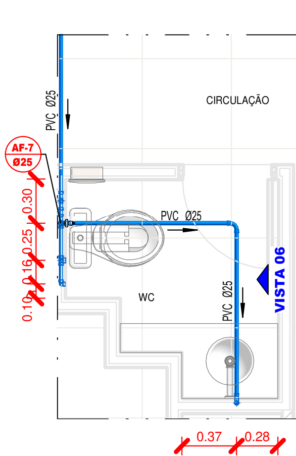
DETALHE 06 - ÁGUA FRIA 1 : 25
